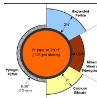
Todos os quatro projetos proporcionam o mesmo nível de proteção térmica (130 Btu/h-ft)
